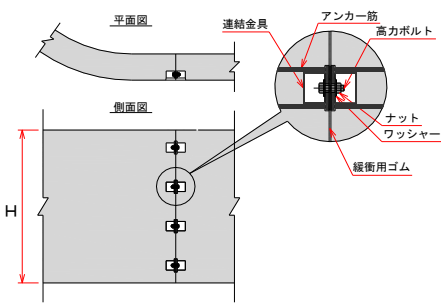
① ボルトによる接合
