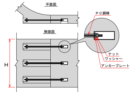
③ PC鋼棒による接合
