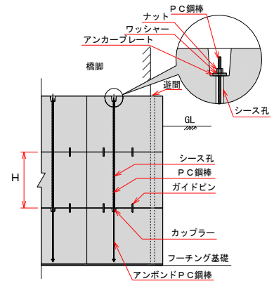
③ PC鋼棒による接合
