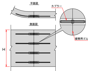
② 機械式継手による接合
