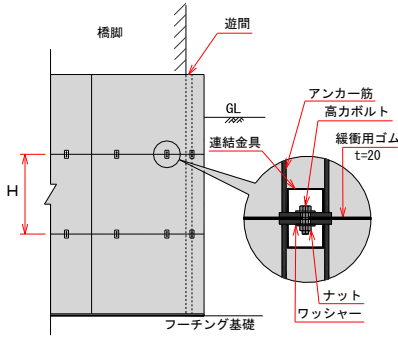
② ボルトによる接合
