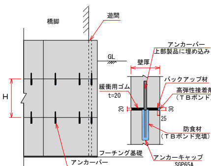
① アンカーバーによる接合
